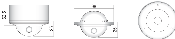
尺寸圖 單位: mm
